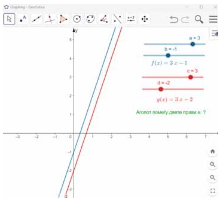
Цртеж 2. Замен однос на две правии ( link ).
