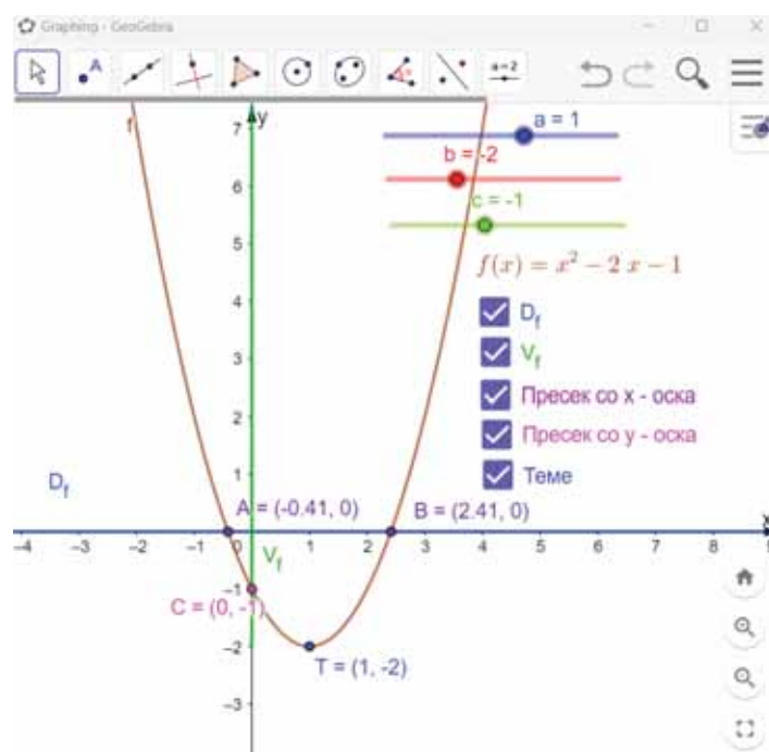
Цртеж 3. График на квадратна функција ( link ).
