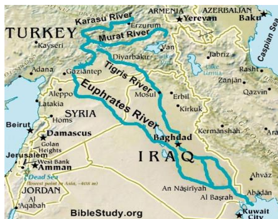
Слика 05, Текот на Реките Тигар и Еуфрат 261
