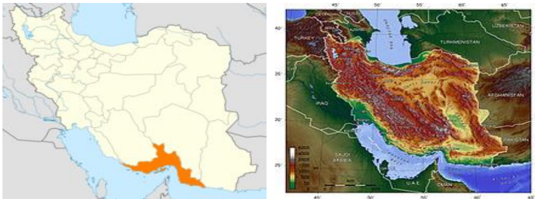
Слика 14, Локација на Хормуз (Hormouz)
