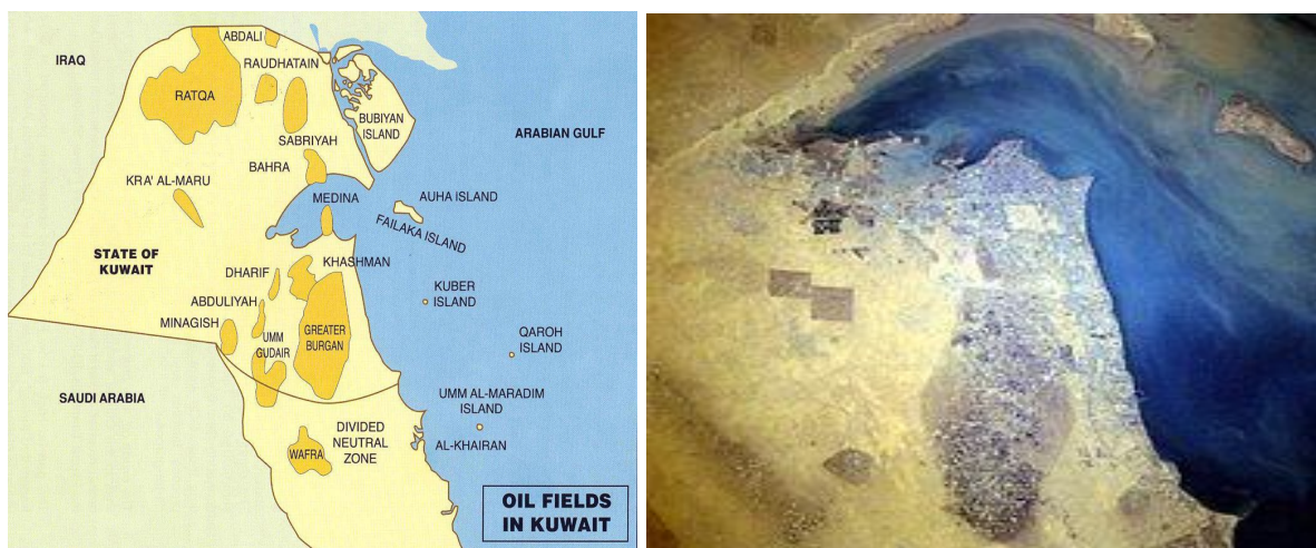
Слика 11, Нафтено поле Бурган 318
