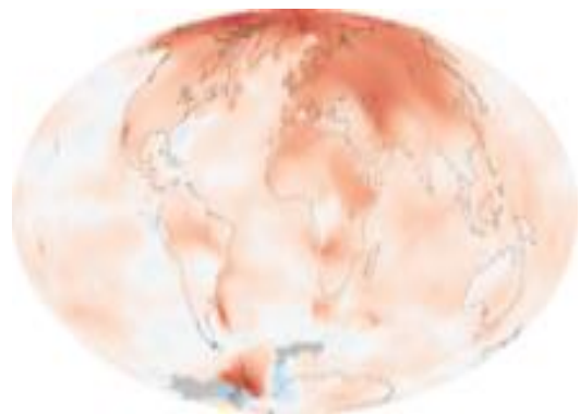
Слика. 23 Зголемување на температурата на Земјата во последните 120 год. 392
