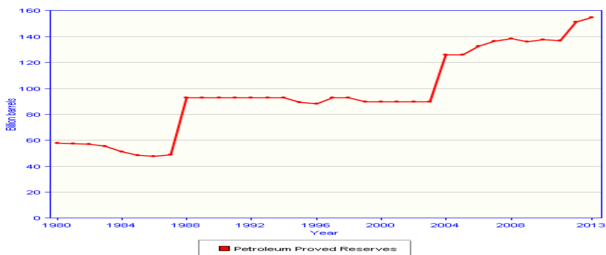
Графикон 8, Утврдени резерви на нафта во Иран 320
