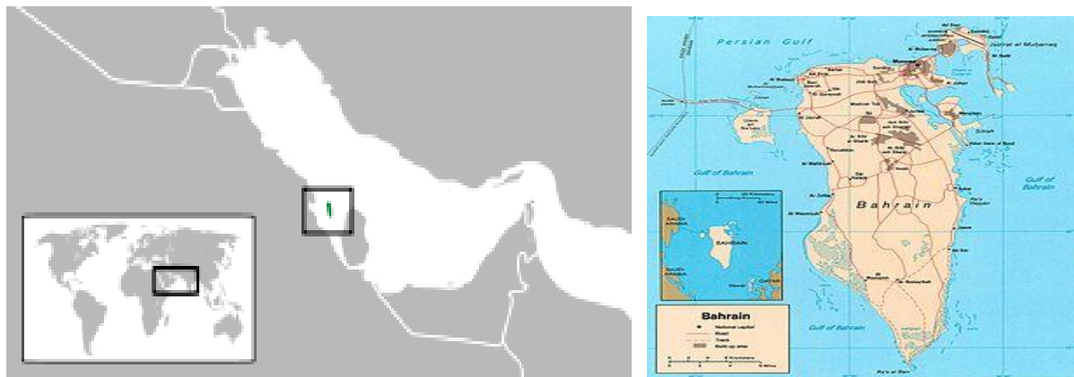
Слика, 19 Локација на Бахреин на Блискиот Исток
