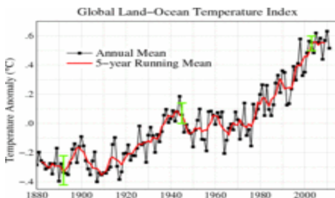
Слика. 23 Зголемување на температурата на Земјата во последните 120 год. 392
