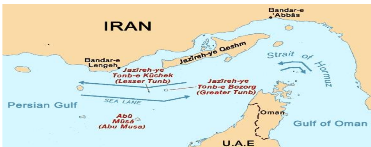
Слика 15, Местоположбата на островите Abu Musa во Персискиот Залив. 361
